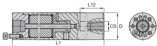
Настраиваемая стальная расточная оправка с внутренним подводом СОЖ.
