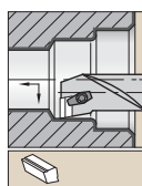
Твердосплавная расточная оправка с внутренним подводом СОЖ.
