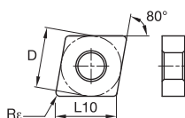
■ CNMG-RBB
