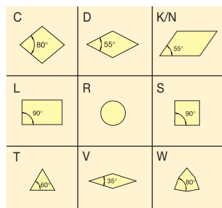
5. Форма пластины
