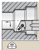
Стальная оправка с внутренней подачей СОЖ
