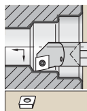
Карбидовая оправка с горловиной и сквозной подачей СОЖ См. стр. A106–A107 с дополнительными сведениями о пластинах
