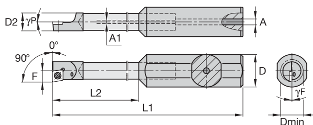
Карбидовая оправка с горловиной и сквозной подачей СОЖ См. стр. A106–A107 с дополнительными сведениями о пластинах
