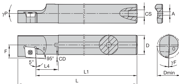
Стальная оправка с внутренней подачей СОЖ См. стр. А108-А109 с дополнительными сведениями о пластинах
