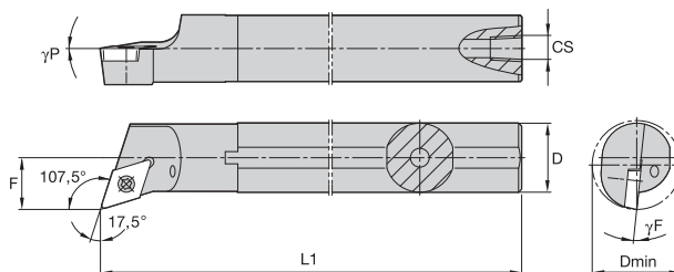
Стальная оправка с внутренней подачей СОЖ См. стр. А112 с дополнительными сведениями о пластинах
