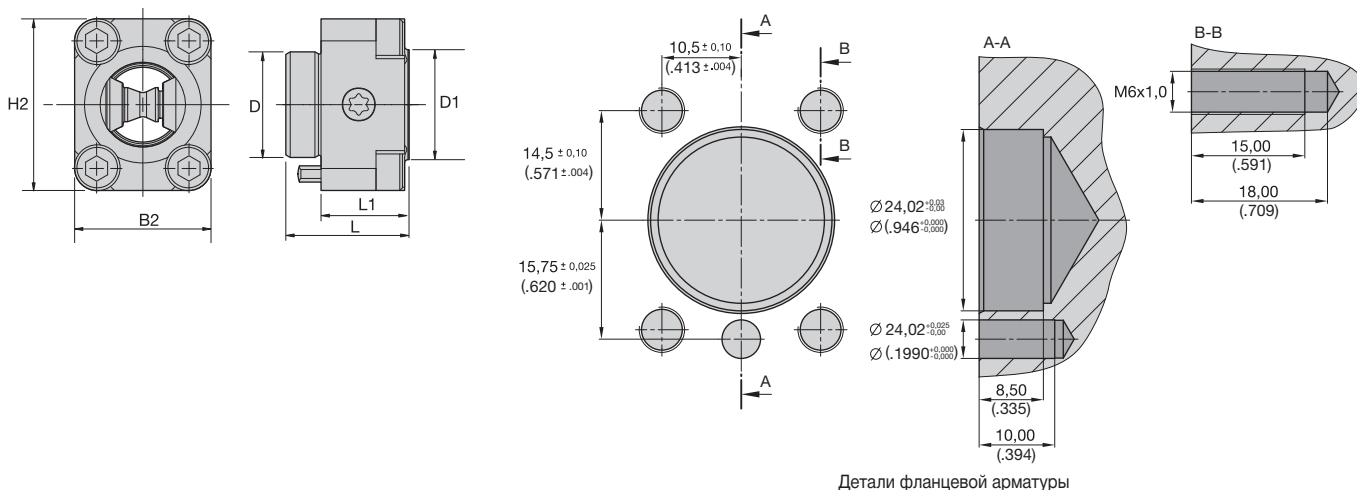
Детали фланцевой арматуры
