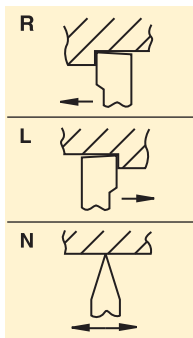
Направление инструмента
